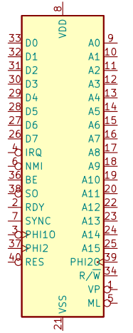
U3 W65C025xxPx-14
