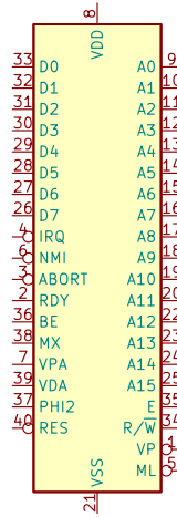
U6 W65C8165xxPx-14
