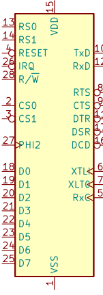
U7 W65C51NxxPLx-14
