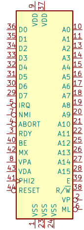
U4 W65C8165xxPLx-14
