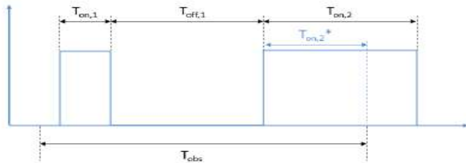
Hình 2 - Minh họa thời gian truyền dẫn lũy kế
