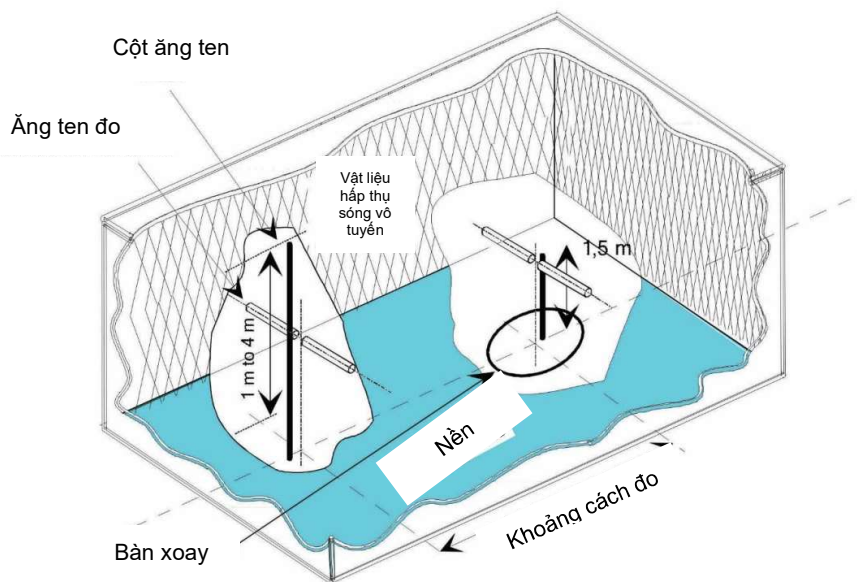
Hình 14 - Phòng bán phản xạ (SAR)
