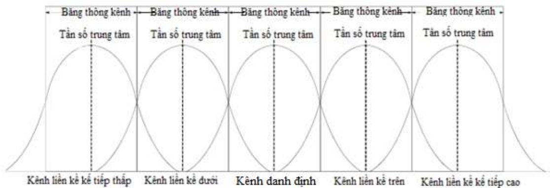
Hình 1 - Định nghĩa các kênh liền kề
