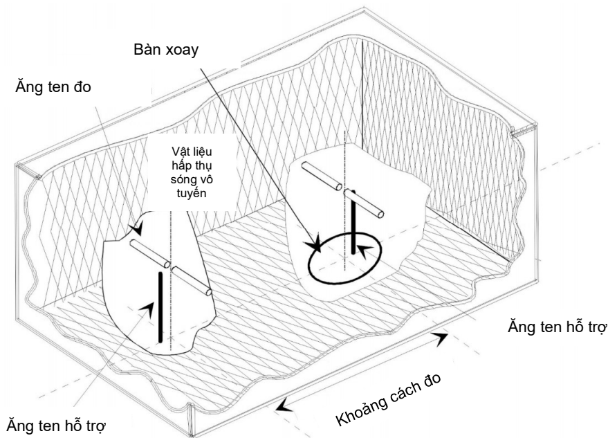
Hình 15 - Phòng không phản xạ (FAR)
