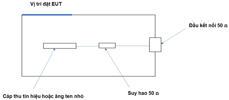
Hình 12 - Phép hộp ghép đo
