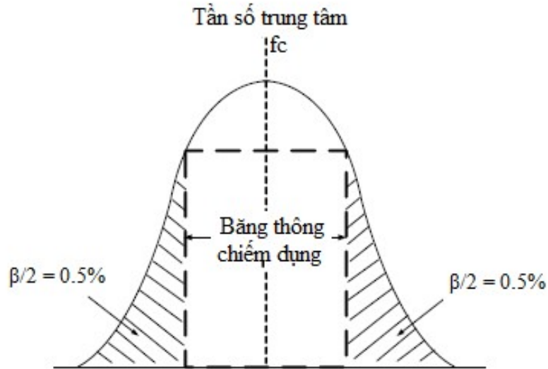
Hình 3 - Băng thông tín hiệu bị chiếm dụng
