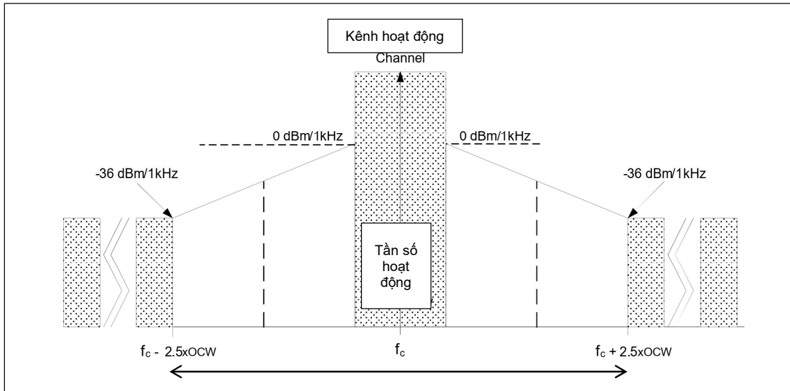
Hình 6 - Miền phát xạ ngoài băng đối với kênh tần số hoạt động với BW tham chiếu
