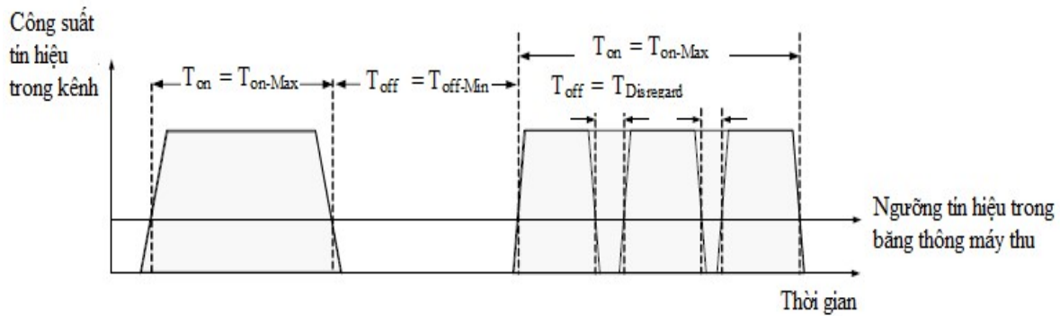
Hình 4 - Các định nghĩa truyền dẫn
