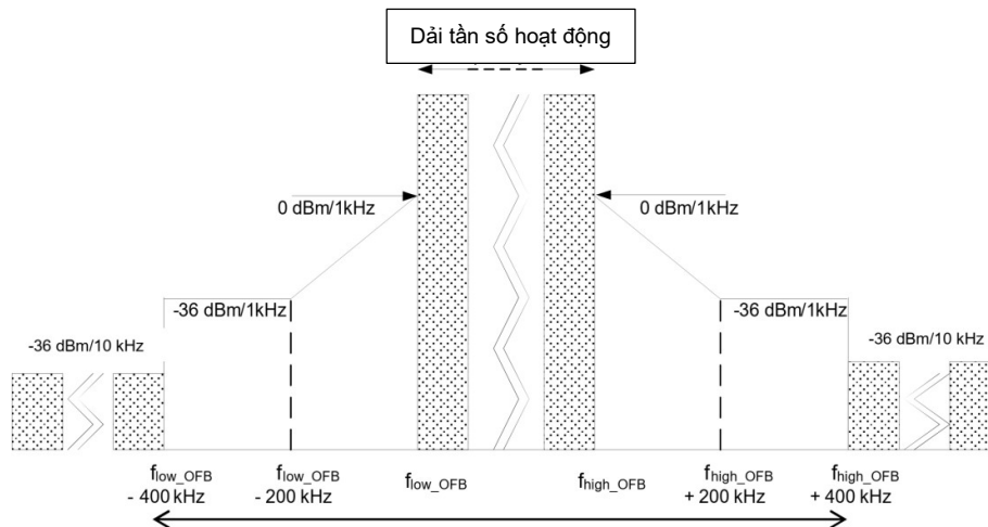
Hình 7 - Miền phát xạ ngoài băng đối cho dải tần số hoạt động với BW tham chiếu
