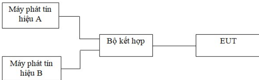
Hình 10 - Sắp xếp đo quá tải đầu vào máy thu
