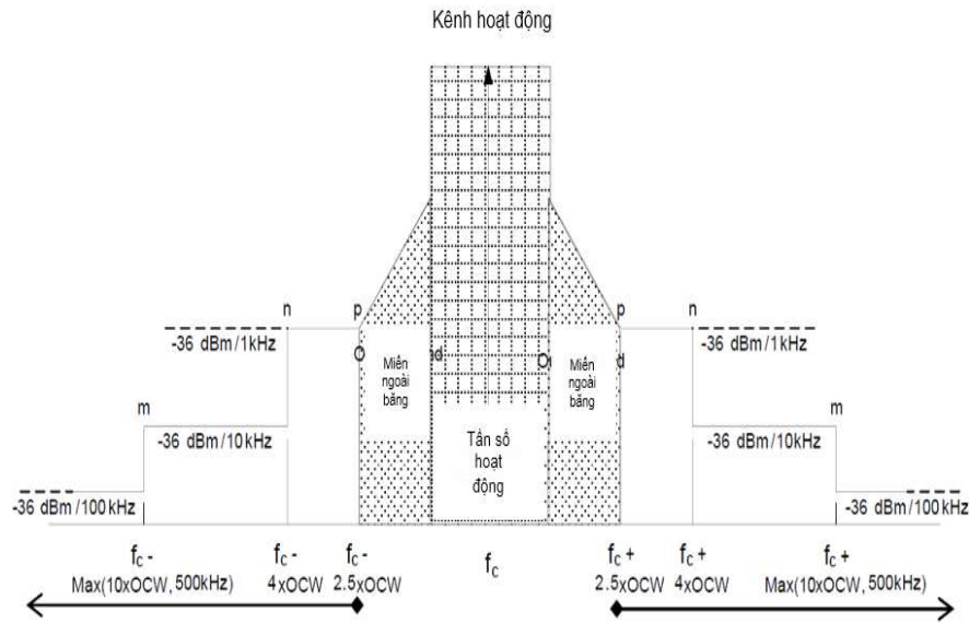
Hình 5 - Mặt nạ phổ cho phát xạ không mong muốn trong miền phát xạ giả với băng thông tham chiếu
