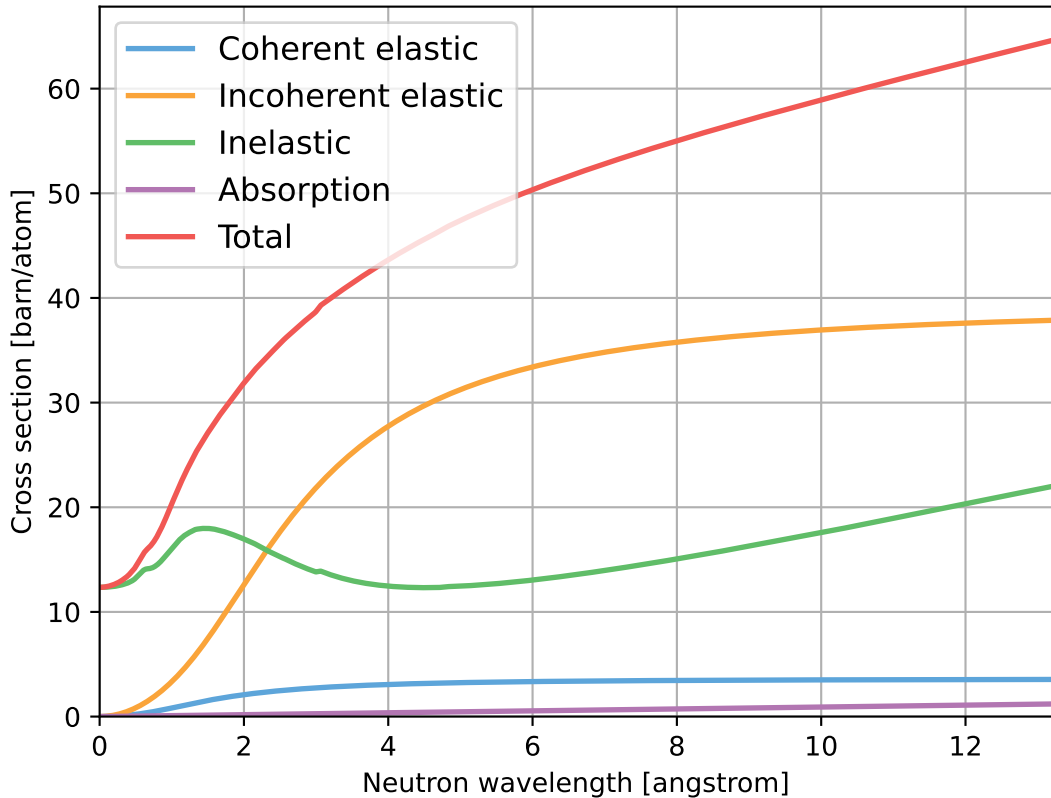
Epoxy_Araldite506_C18H20O3.ncmat
