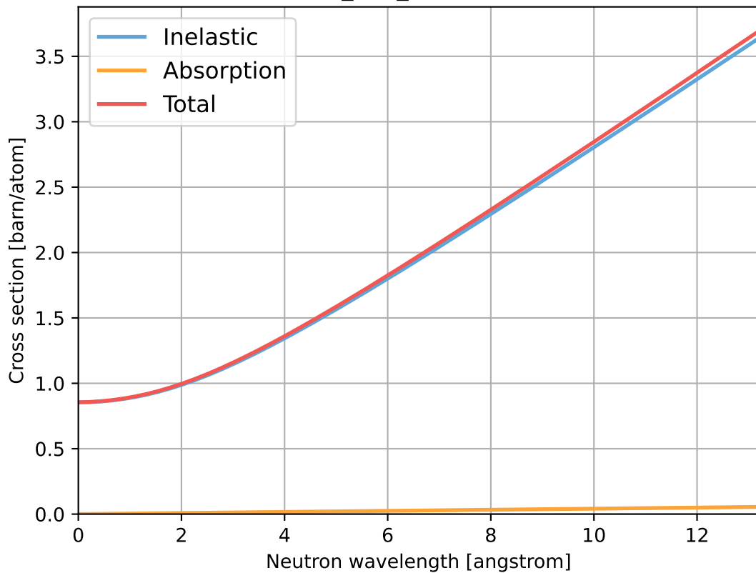
He_Gas_STP.ncmat
