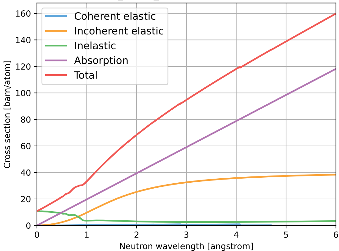
LiH_sg225_LithiumHydride.ncmat
