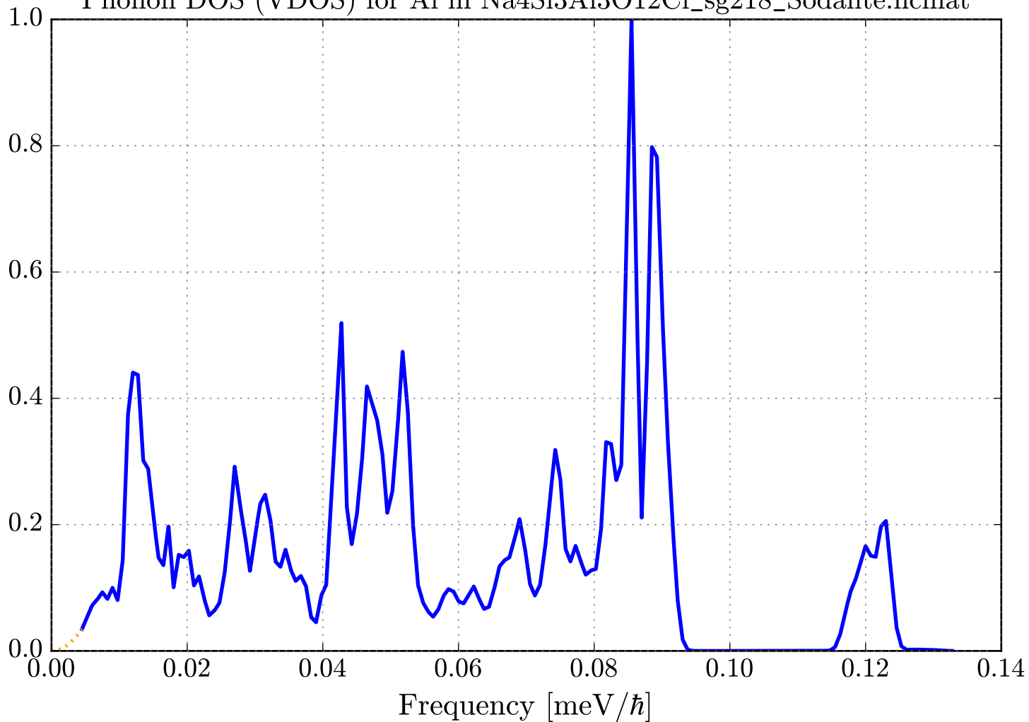
Phonon DOS (VDOS) for Al in Na 4 Si 3 Al 3 O 12 Cl_sg218_Sodalite.ncmat
