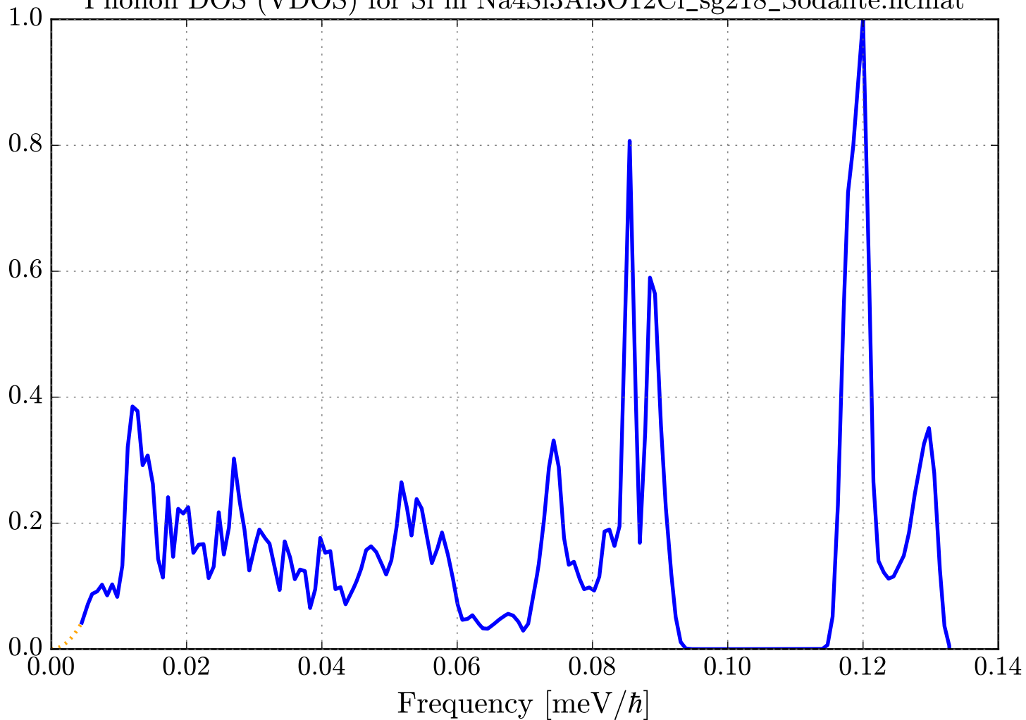
Phonon DOS (VDOS) for Si in Na 4 Si 3 Al 3 O 12 Cl_sg218_Sodalite.ncmat
