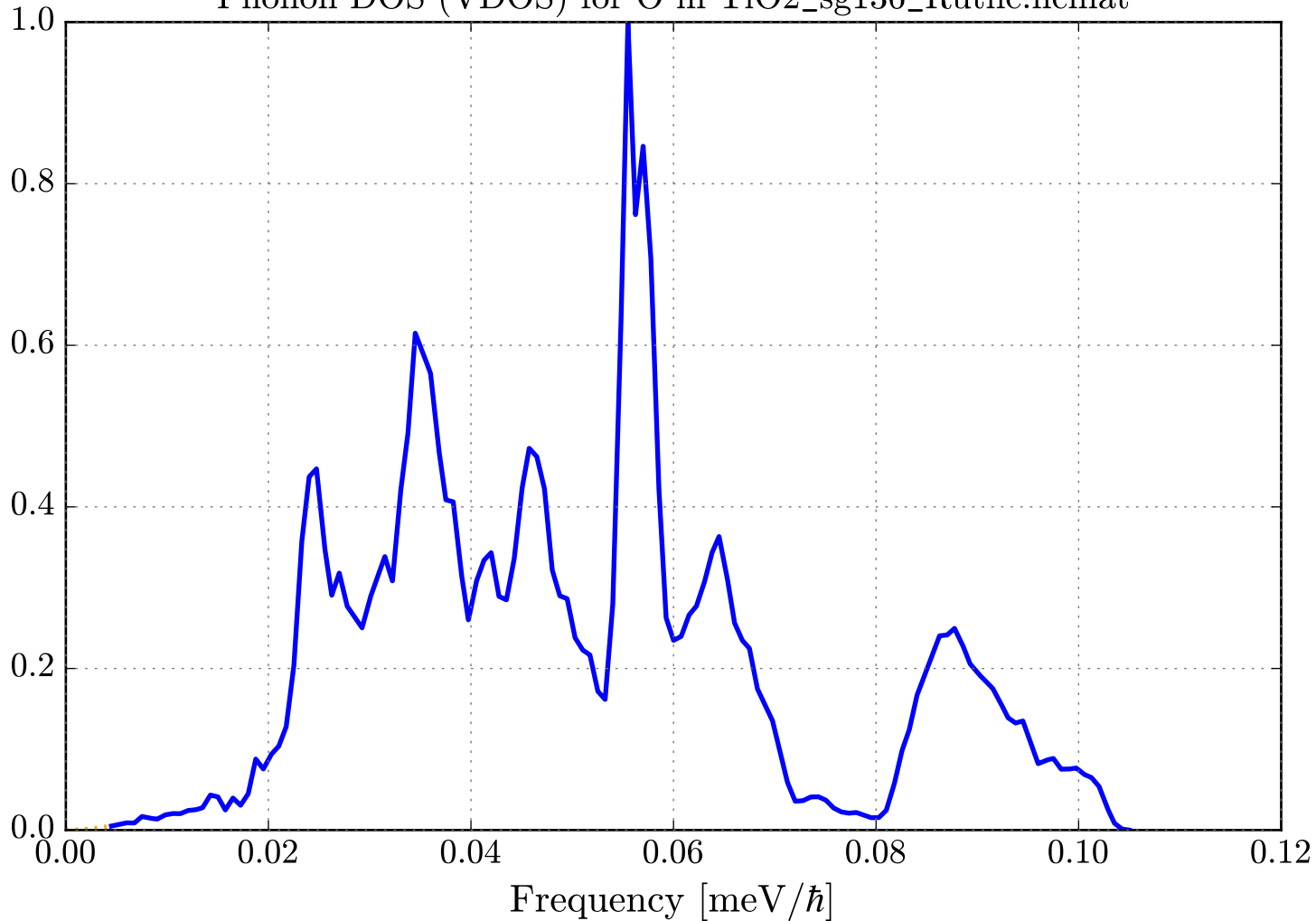
Phonon DOS (VDOS) for O in TiO2_sg136_Rutile.ncmat
