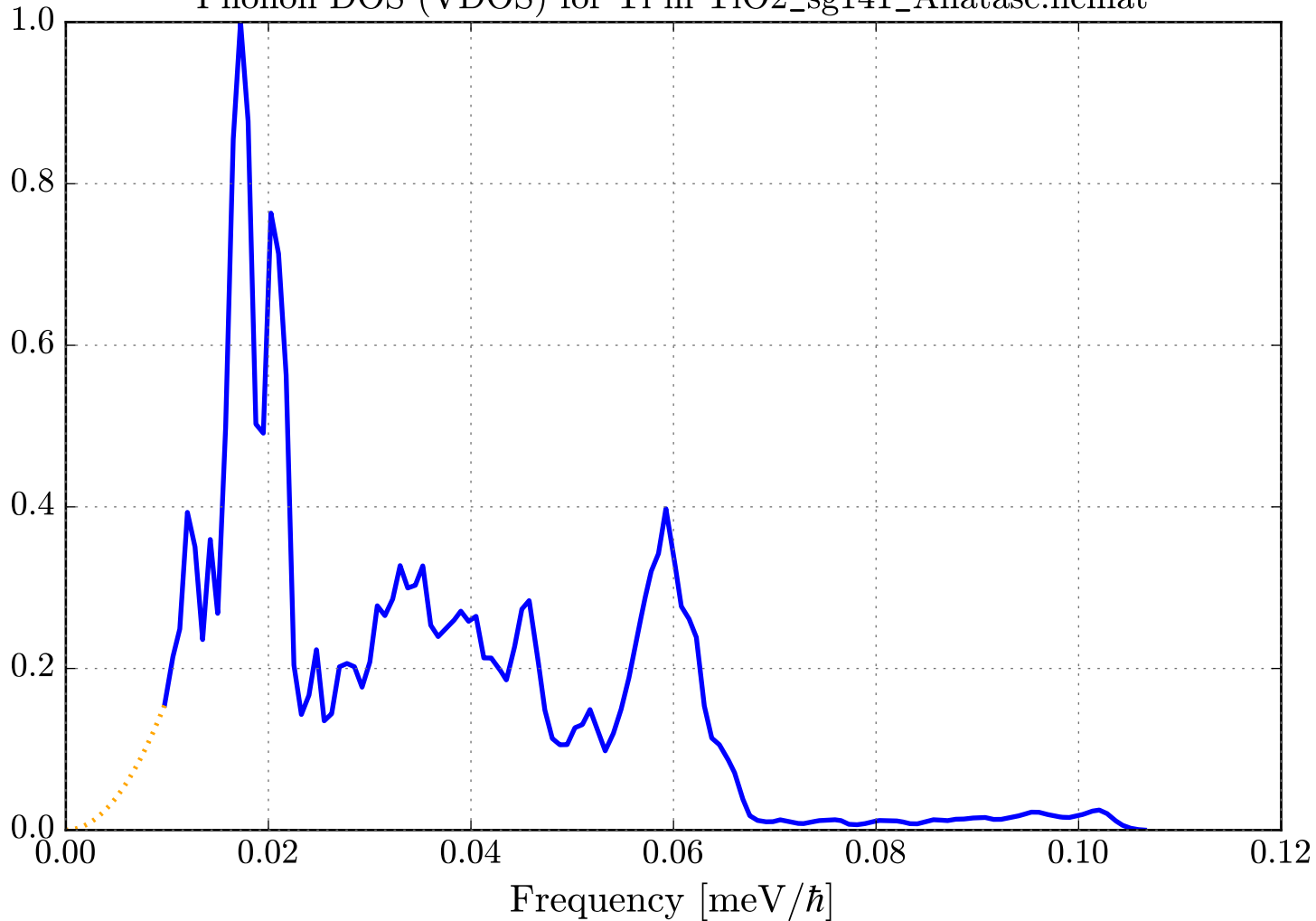
Phonon DOS (VDOS) for Ti in TiO2_sg141_Anatase.ncmat
