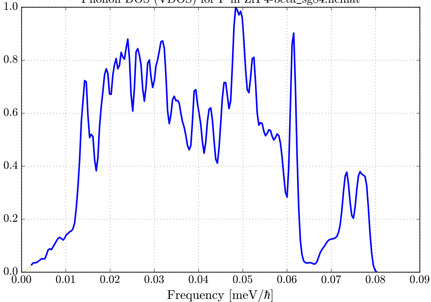
Phonon DOS (VDOS) for F in ZrF4-beta_sg84.ncmat
