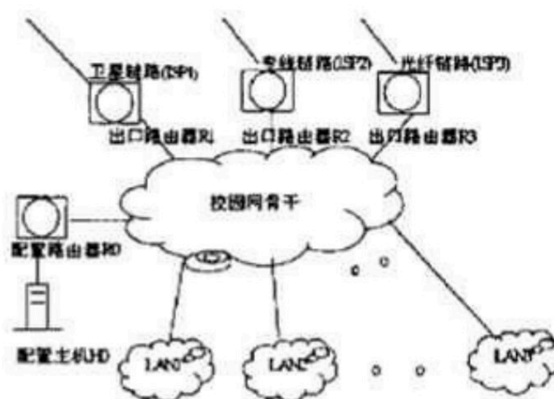
图 1 动态路由学习方式的 IP 封堵系统连接示意图
