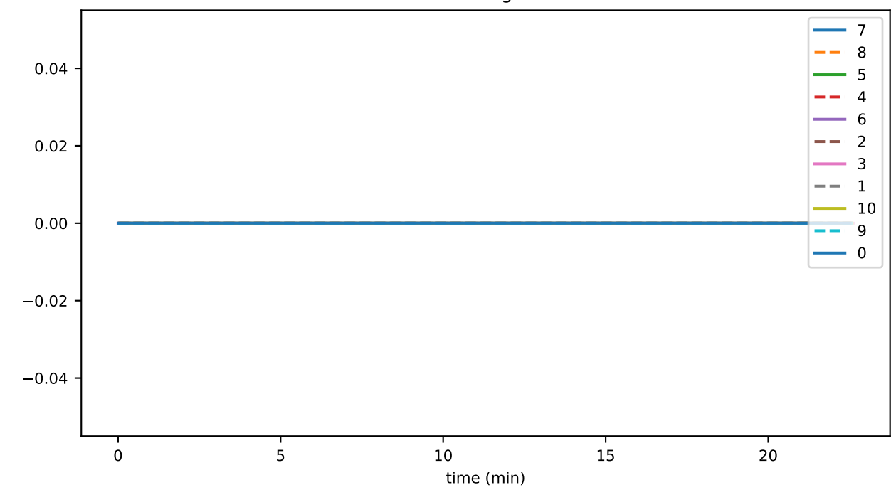
TtIDig
