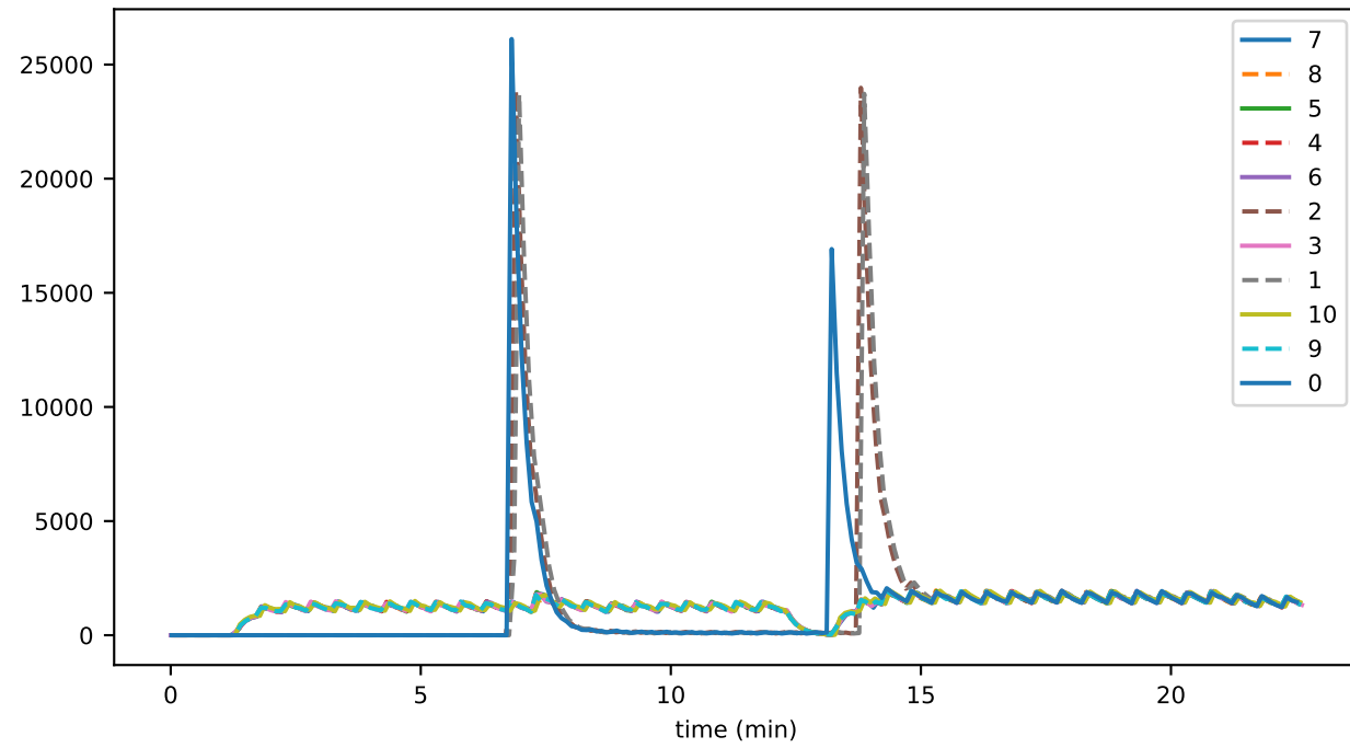
vmUpdate
