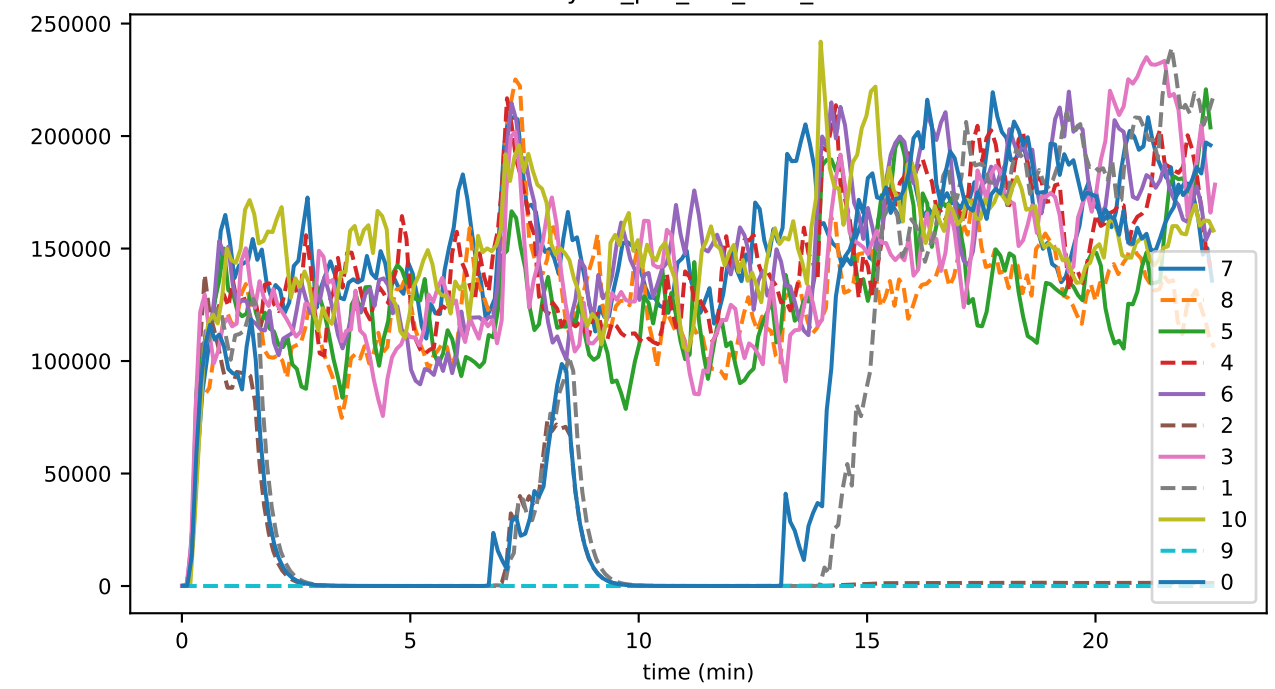
bytes_per_sec_sent_09
