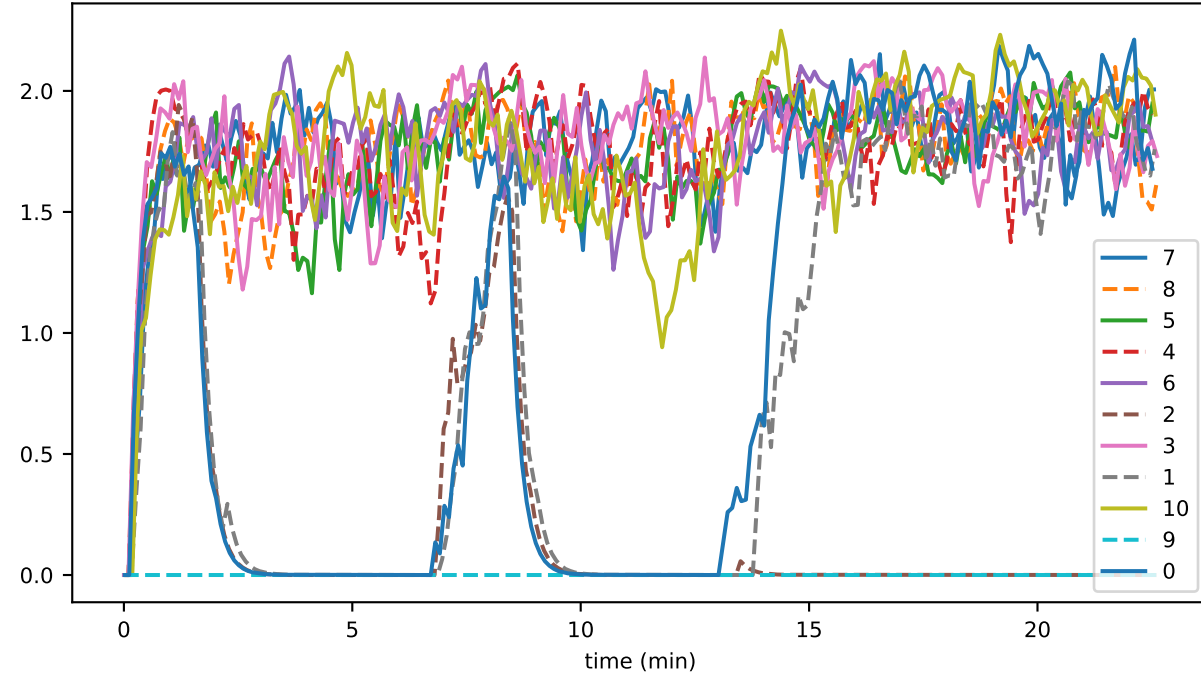
tipsetParent9
