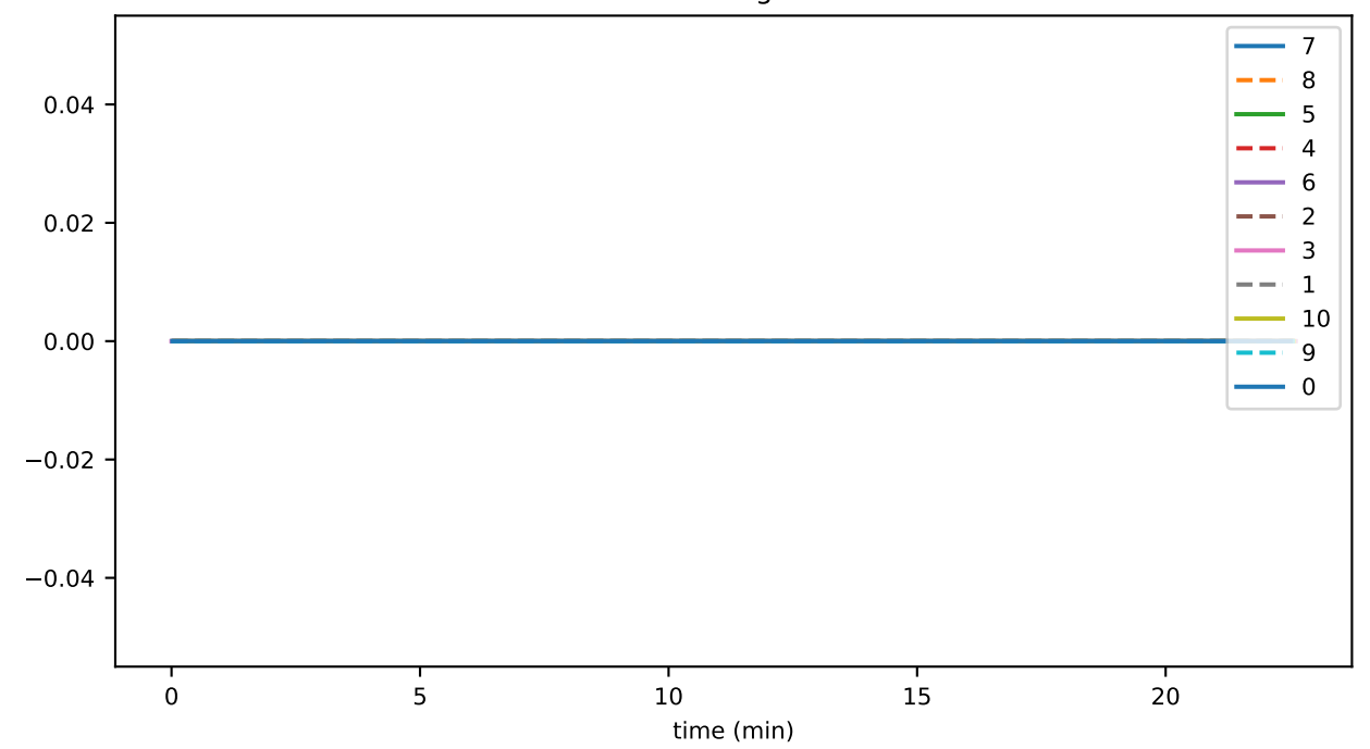
TtISig
