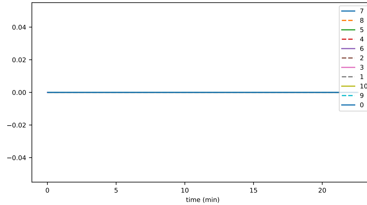
fcqRemoveExecMicroSec
