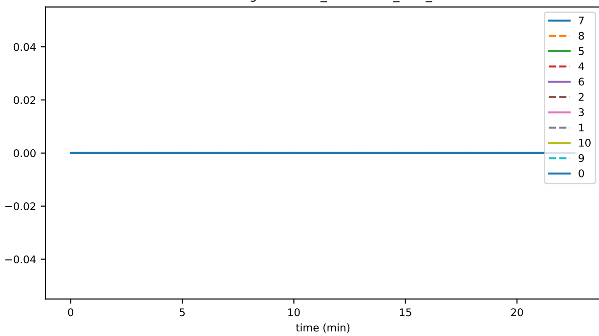
StateGarbageCollector_unhandled_task_count
