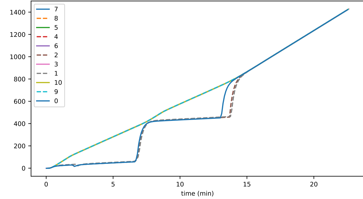
roundSup
