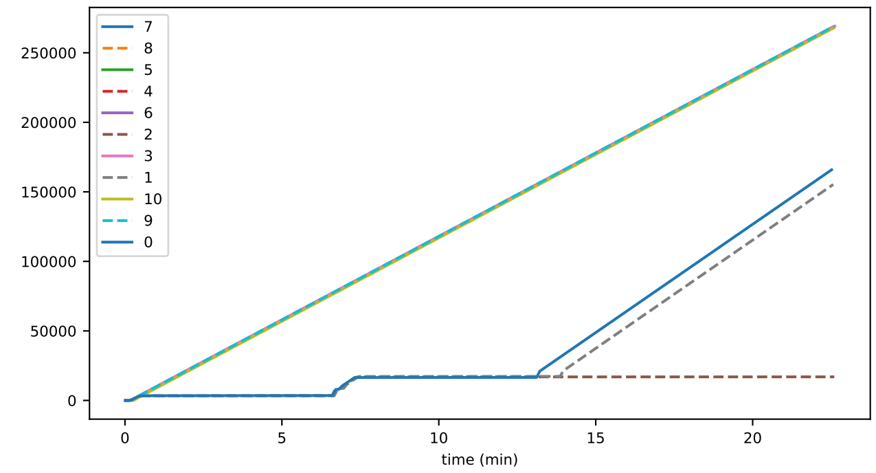
TtIDig
