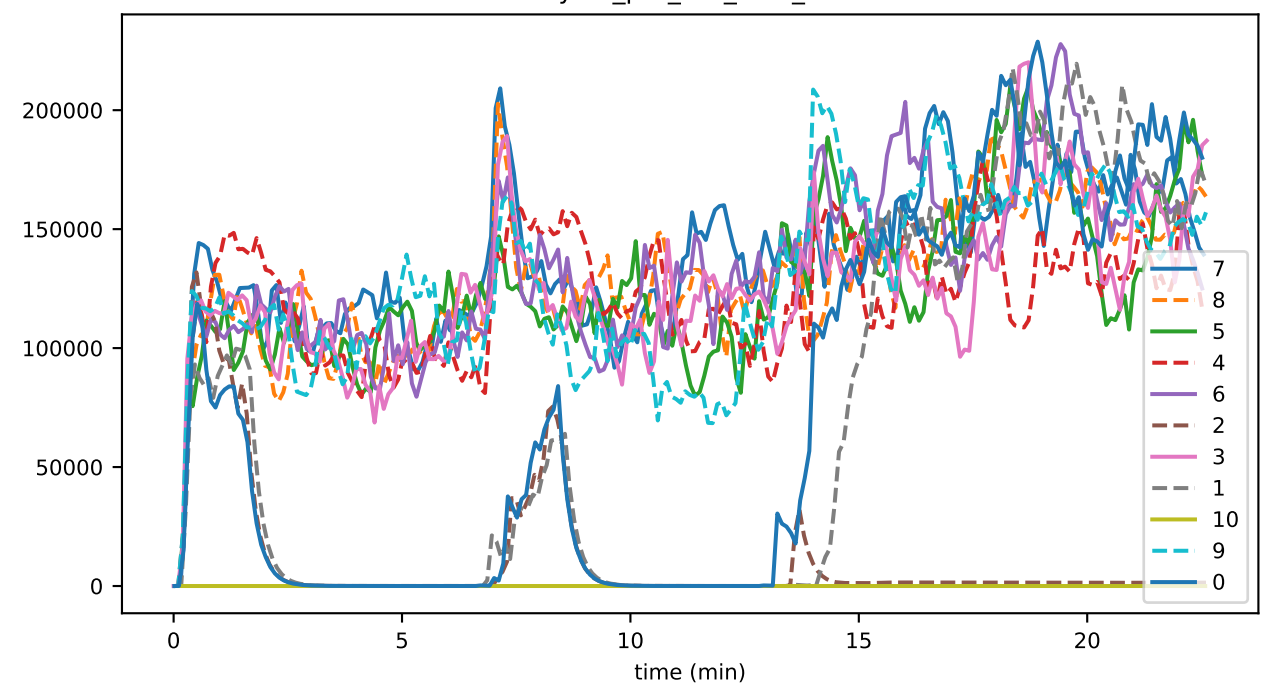
bytes_per_sec_sent_10
