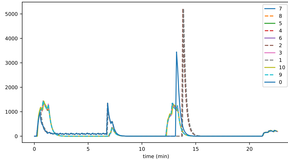
vmUpdate
