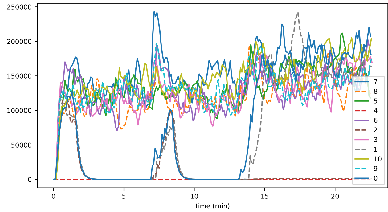
bytes_per_sec_sent_06
